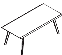
EW80 W2000*D950*H760(mm)
