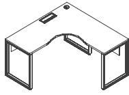
DL65(L/R)-2.GJ W1400*D1400*H750 W1500*D1500*H750 W1600*D1600*H750
