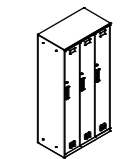
DC94.18 W900*D515*H1822
