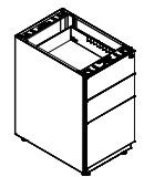
DC93.07 W397*D590*H725
