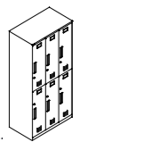
DC95.18 W900*D515*H1822
